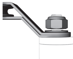
Instalación correcta PATROLANG en soporte TOWER - TOWER22 - TOWERA2
